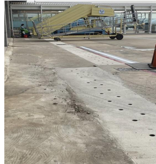
3 號-6 號停機坪登機廊道與停機坪 PC 鋪面交界處(改善前)圖-2
